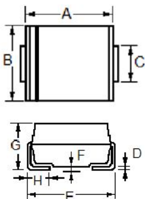
DO-214AB (SMC)
