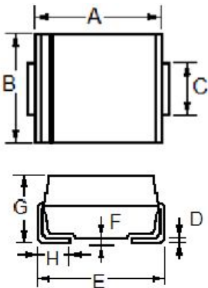
DO-214AB (SMC)
